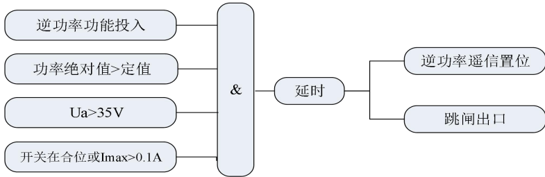
图 5.6 逆功率逻辑图
