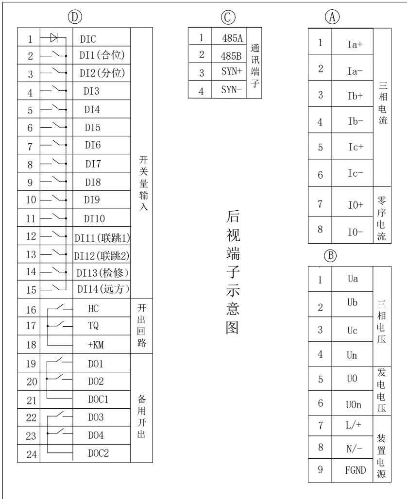
图 6.1 后视端子图
