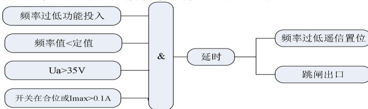
图 5.4 频率过低逻辑图
