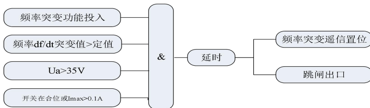
图 5.5 频率突变逻辑图
