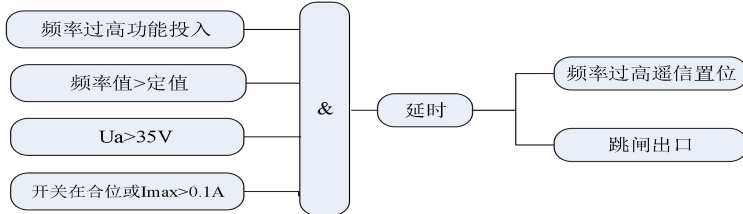
图 5.3 频率过高逻辑图
