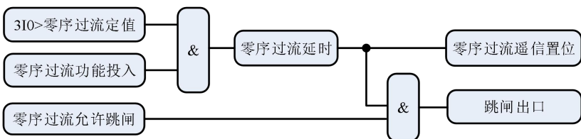
图 5.10 零序过流逻辑图
