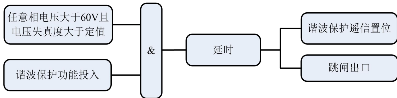
图 5.7 谐波保护逻辑图
