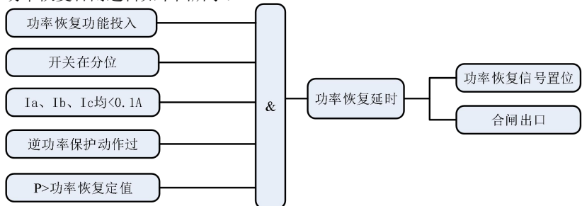
图 5.13 功率恢复合闸逻辑图
